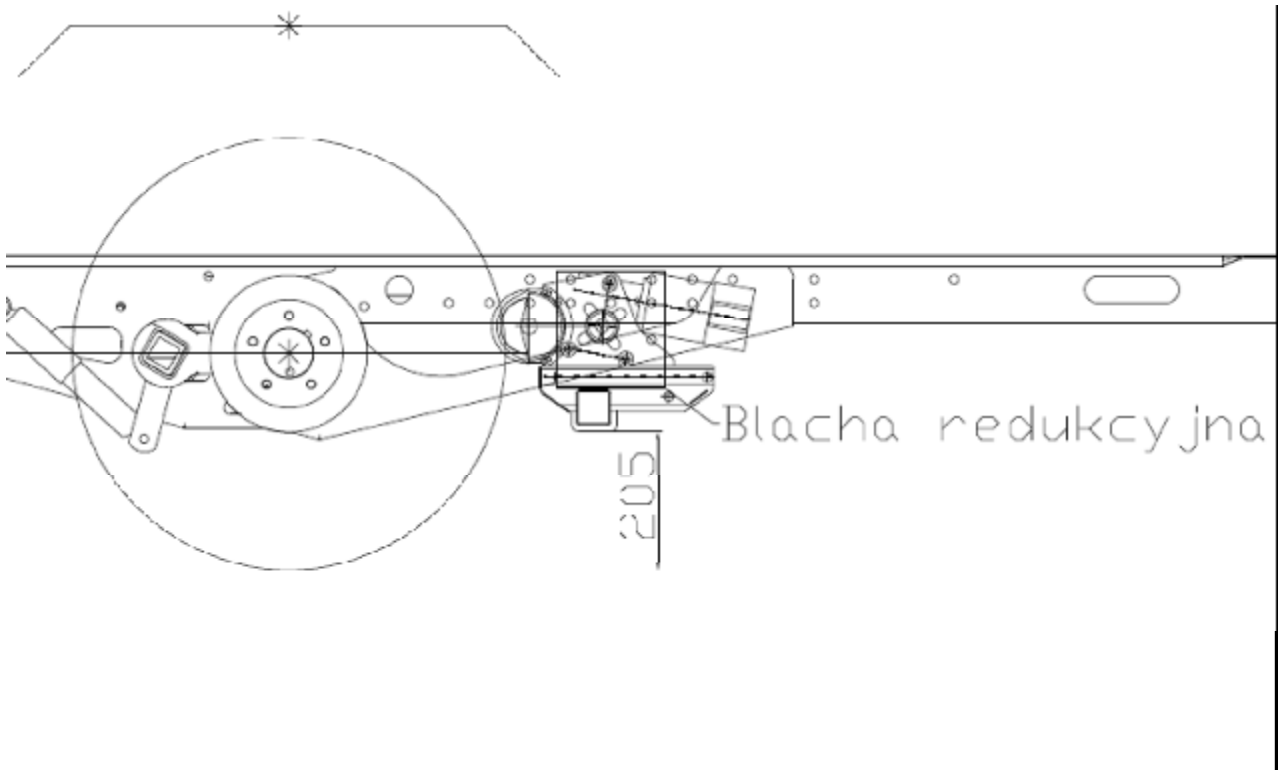
Rysunek 2 (widok z zewnątrz, lewa strona).
