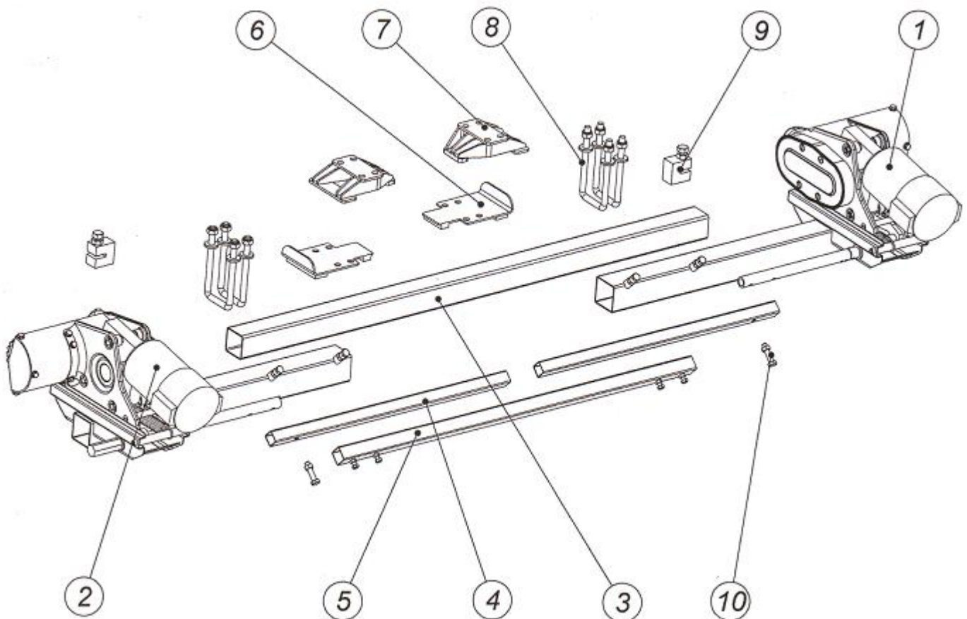
Rysunek 4 Rysunek złożeniowy urządzenia Smart Drive Single.
